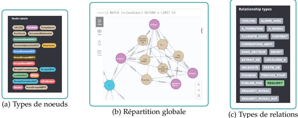
Figure 3.10 – Lecture conjointe des noeuds et relations Neo4j mobilisés par le matching
